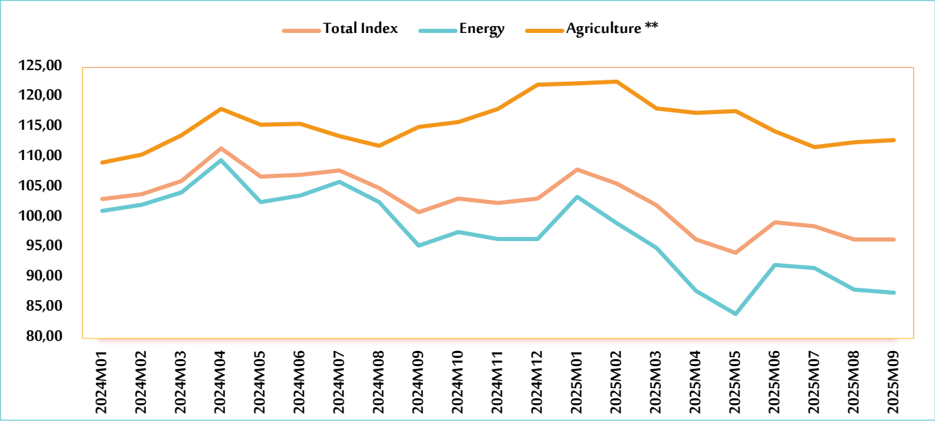
Graphique 1 : évolution des cours de matières premières
